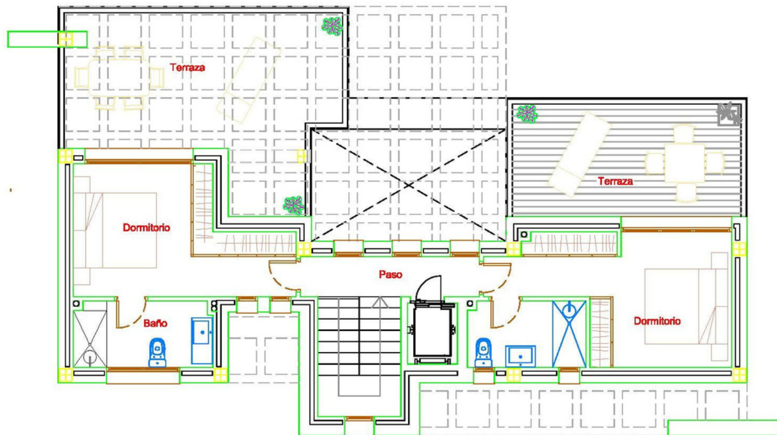
PLANTA ALTA VIVIENDA UNIFAMILIAR AISLADA Y PISCINA C/ MARGALLÓ, Nº 1-3. PARCELA 1
