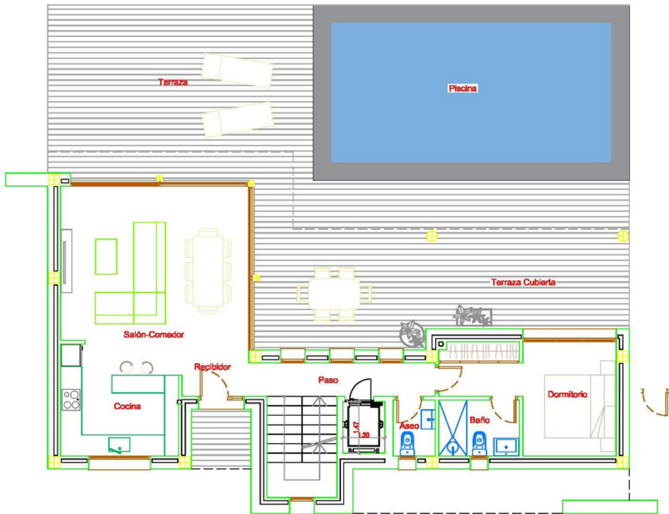
PLANTA BAJA VIVIENDA UNIFAMILIAR AISLADA Y PISCINA C/ MARGALLÓ, N° 1-3. PARCELA 1
